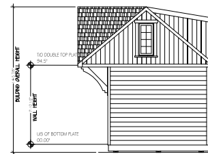
10 RIGHT ELEVATION SCALE: 1/4" = 1'-0"
