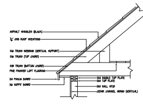
14 TRUSS DETAIL SCALE: 1" = 1'-0"
