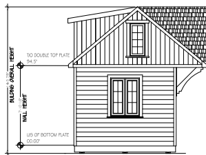
8 LEFT ELEVATION SCALE: 1/4" = 1'-0"
