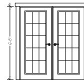
20 DD6 ELEVATION SCALE: 3/8" = 1'-0"
