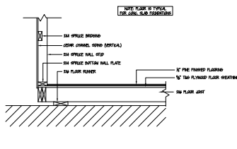
13 FLOOR DETAIL SCALE: 1" = 1'-0"
